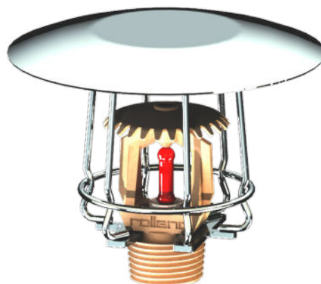
Coupelle Ø150
