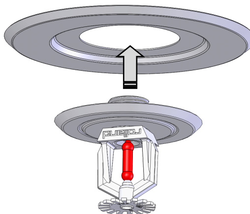
Assembly with simple escucheon
